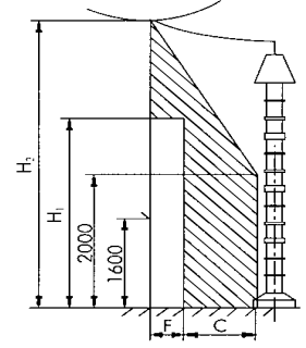
Şekil-7 Yere konulan normal çiti bulunan aygıtlarda koruma alanı
