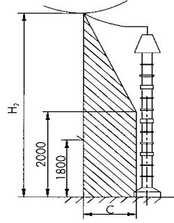
Şekil-6 Yere konulan ve geçitsiz normal çiti bulunan aygıtlarda koruma alanı
