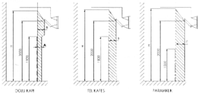
Şekil-2 Açık bağlama tesislerinde koruma alanları (taranmış bölümler) ve en küçük yükseklikler. Şekil üzerindeki değerler yalnızca 30 kV'a kadar geçerlidir. 45 kV ve daha büyük gerilimler için Şekil-4'e bakınız. Şekil-2'deki harfler, Çizelge-1'deki açıklıkları göstermektedir.
