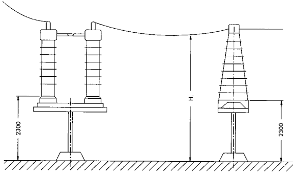
Şekil-3 Tesis içerisinde çitle çevrilmemiş yürütülen yüzeyler üzerindeki iletkenlerin yerden yükseklikleri (Çizelge-3'e göre).
