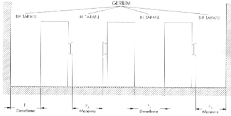
Şekil-1 Hücresel yapıların tel kafes kapı ve dolu duvar olması durumunda geçit genişlikleri
