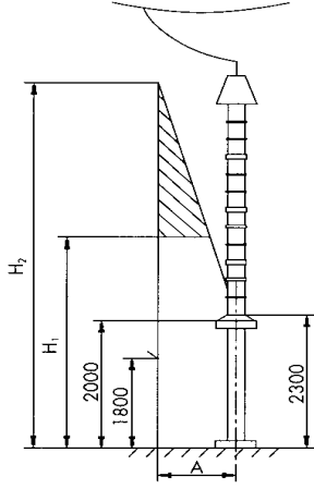
Şekil-5 Dayanak (mesnet) ve geçitli üzerindeki aygıtlarda koruma alanı
