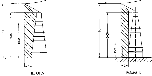
Şekil-4 Tesis içerisindeki koruma alanı ve en küçük yükseklik (H1)
